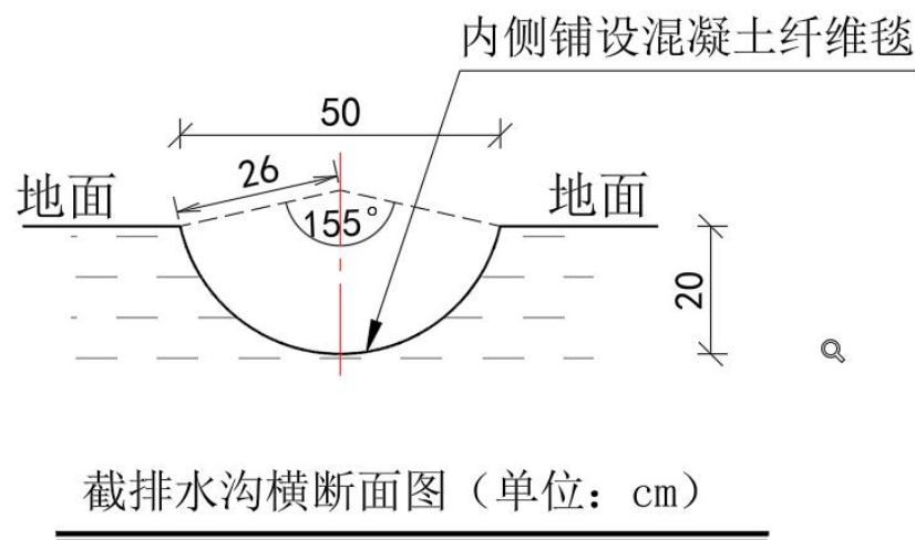
图 5.2-1 截水沟断面示意图
